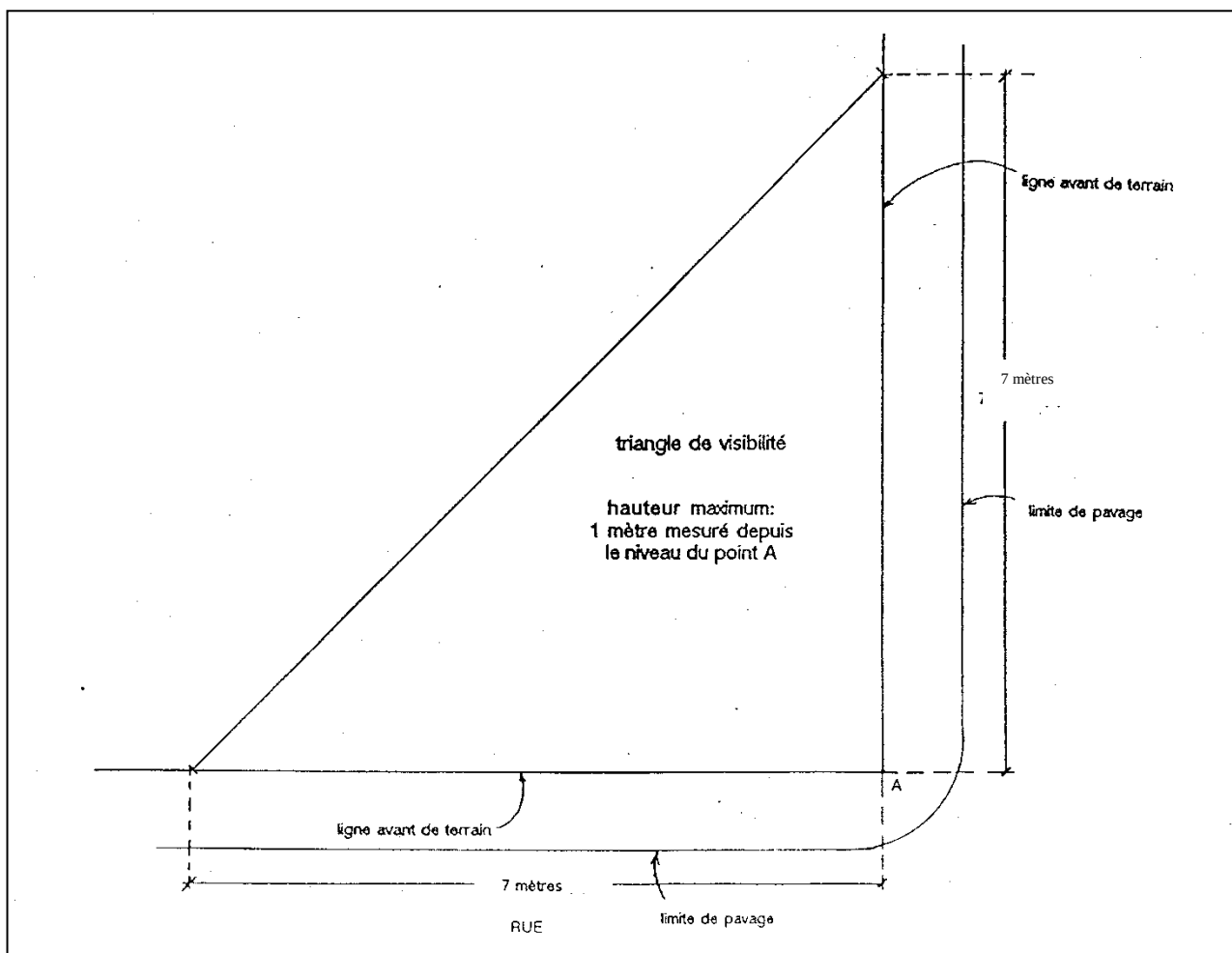
Figure 2 : Visibilité aux carrefours
